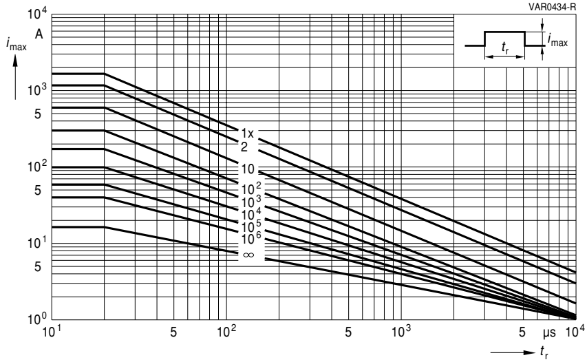
SIOV-S07K50 ... K320E2
