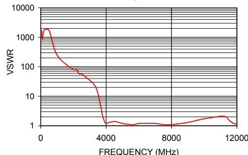
VHF-3800+ VSWR
