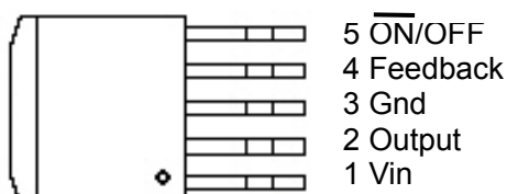
TO263-5L
