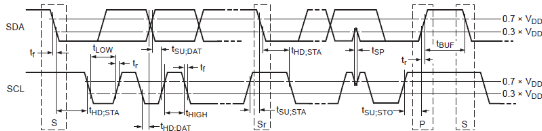
图 1-1 I 2 C 接口时序图
