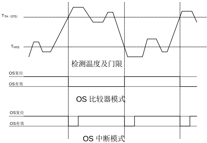
图 2-1 OS 输出与温度关系 (假定每次错误队列数量都满足，且中断模式下每次触发后均被复位)
