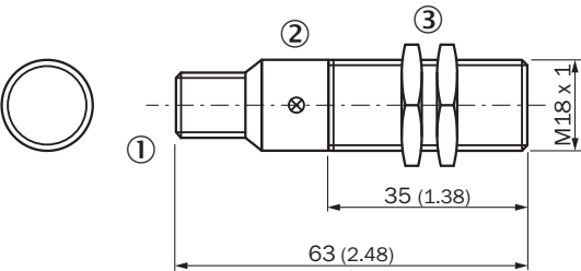
尺寸图 (尺寸单位: mm)
