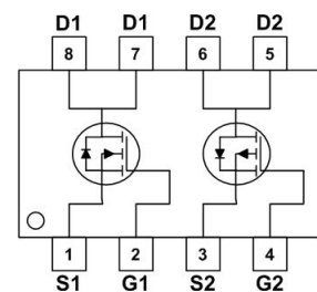
SOP8
