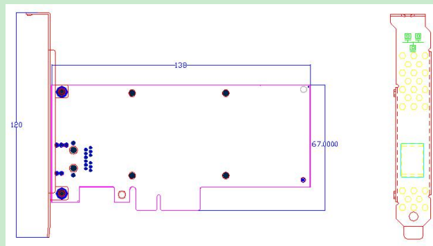
产品结构图
