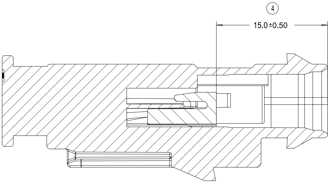
SECTION V-V
