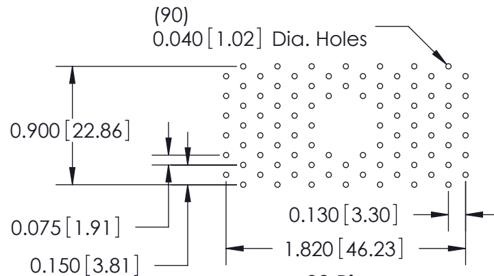
90 Pin P.C. Tail Layout
