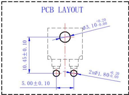
PCB 安装孔示意图
