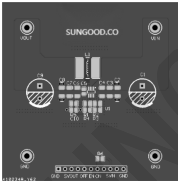
Top Layer
