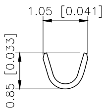
SEC:B-B
