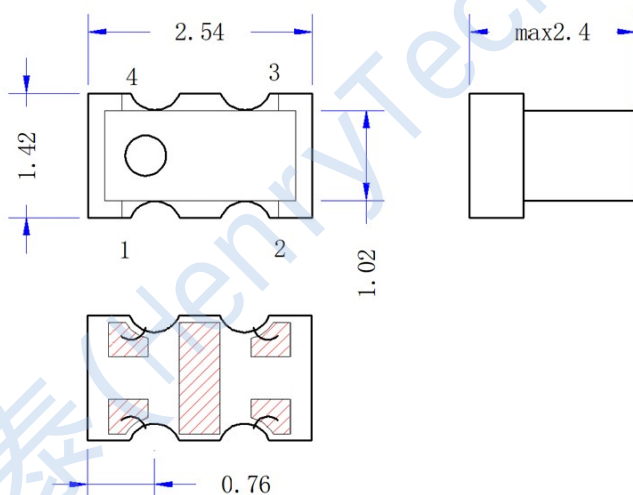
外形结构图 (mm)
