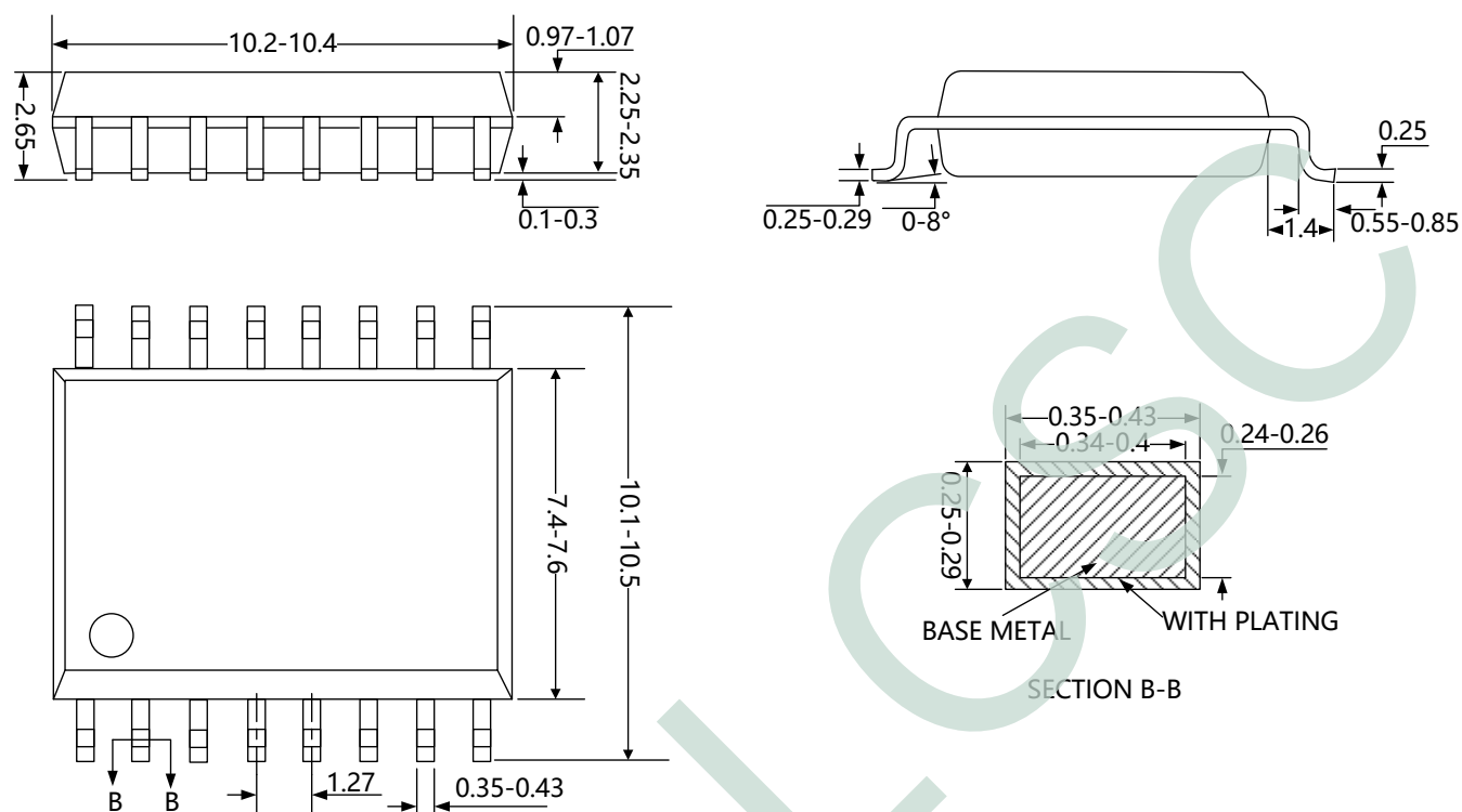
Fig. C1. SOW-16
