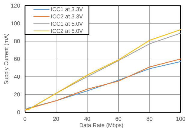
Fig. 8.1. 供电电流 vs. 数据率 (0 pF 负载, 室温)
