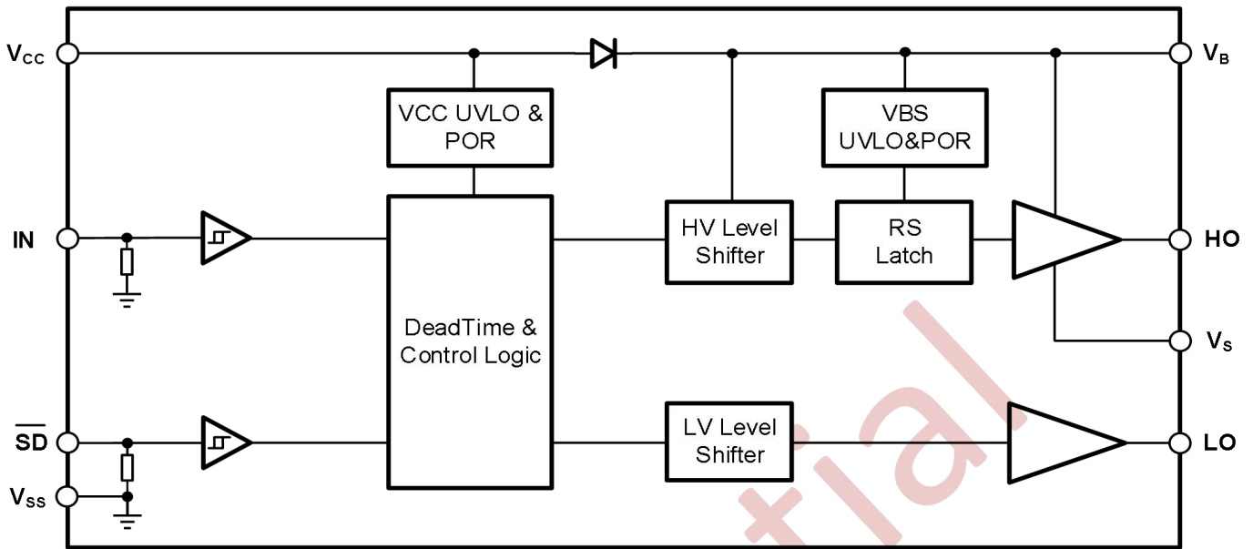
图 10-1 NSG2027 功能框图
