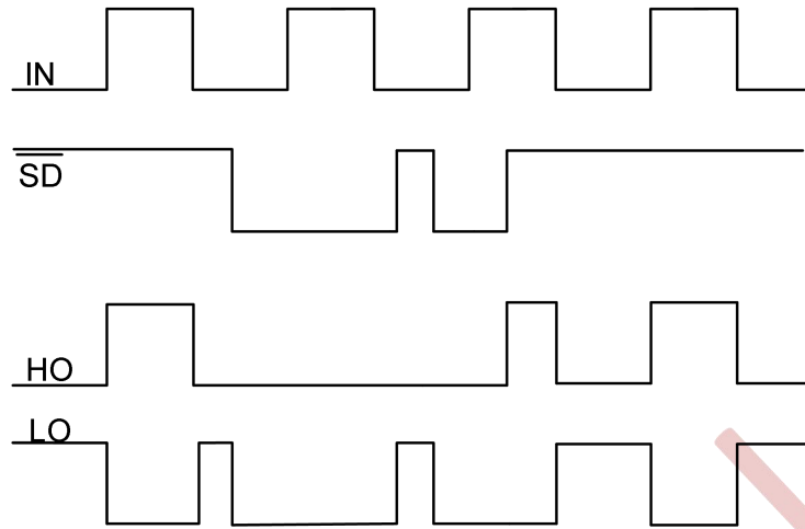
图 9-1 NSG2027 输入输出时序波形
