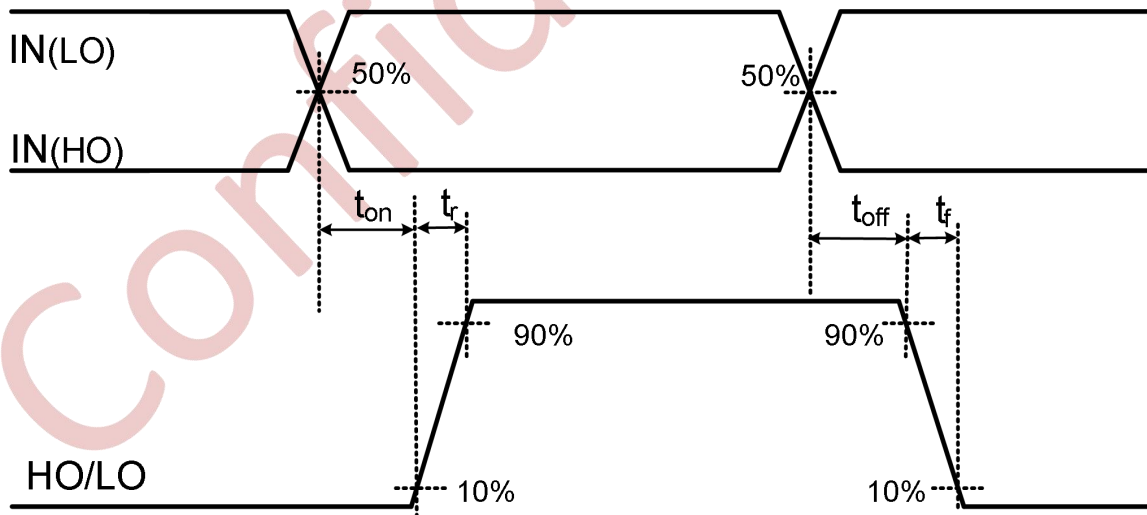
图 9-2 传输延时波形定义
