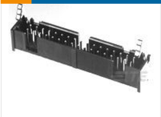
TE Part #1-1761606-1 IDC LOW PRO HDR 34P VERT LG LAT BLK
