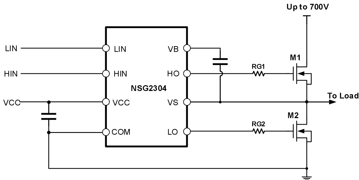
图 10-2 NSG2304 典型应用电路图
