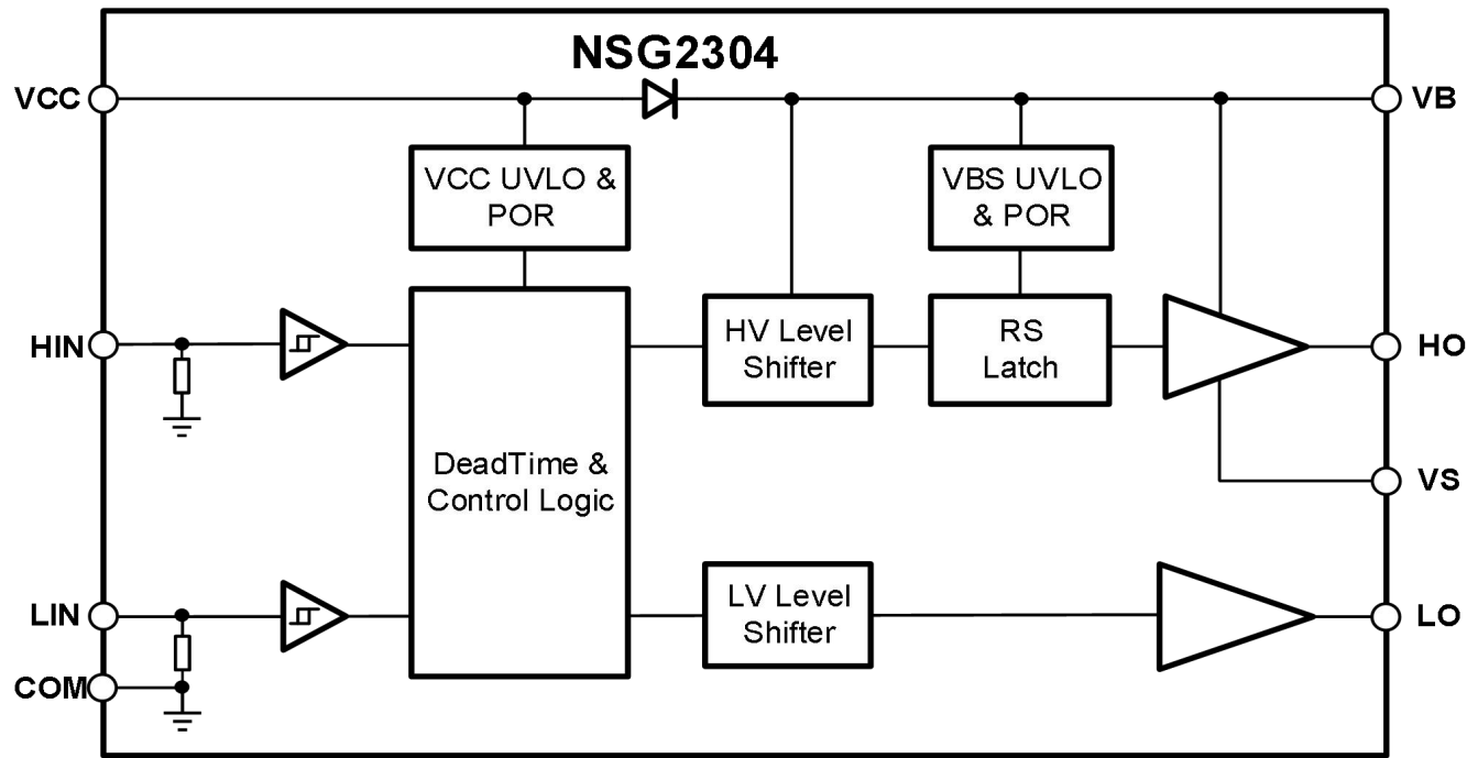
图 10-1 NSG2304 的功能框图
