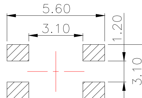
PCB.焊接图
