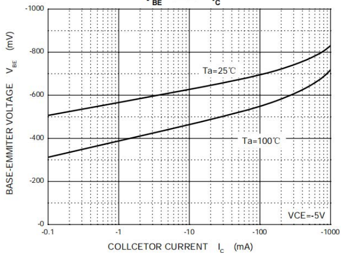
V_{BE} — I_c
