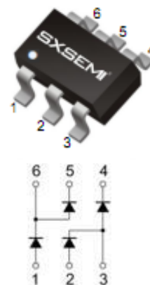
SOT-363
