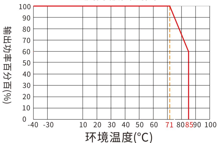
温度降额曲线图
