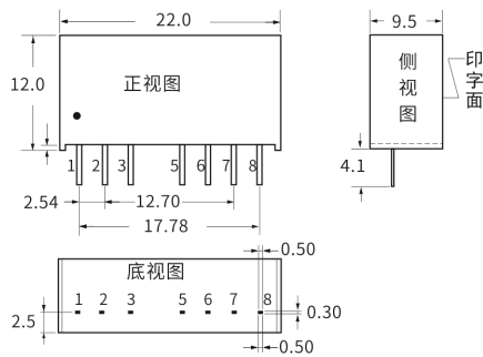
1) 外观尺寸 (单位: mm, 公差: xx \pm 0.25 )
