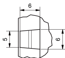
E (2 : 1)
