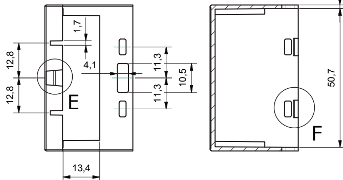
F (2 : 1)
