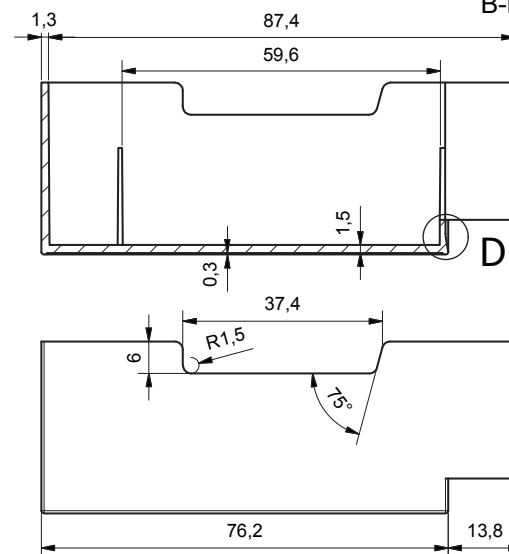
B-B (1 : 1)
