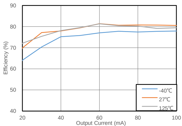
图 8.10 转换效率 vs 输出电流 (CMP6503S+CMT6870N, 3.3V to 3.3V, SEL=VDD)
