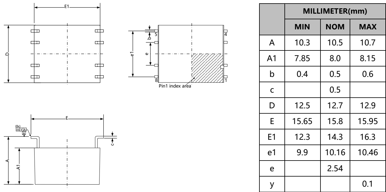
Fig. D.1 SMD-8 器件外形 (所有尺寸单位为 mm)
