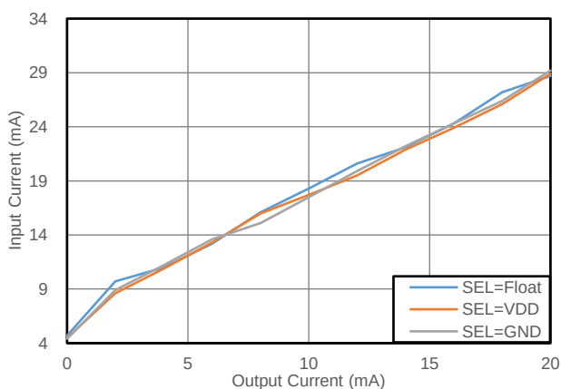
图 8.12 轻载原边供电电流 (CMP6503S+CMT6870N, 3.3V to 3.3V)
