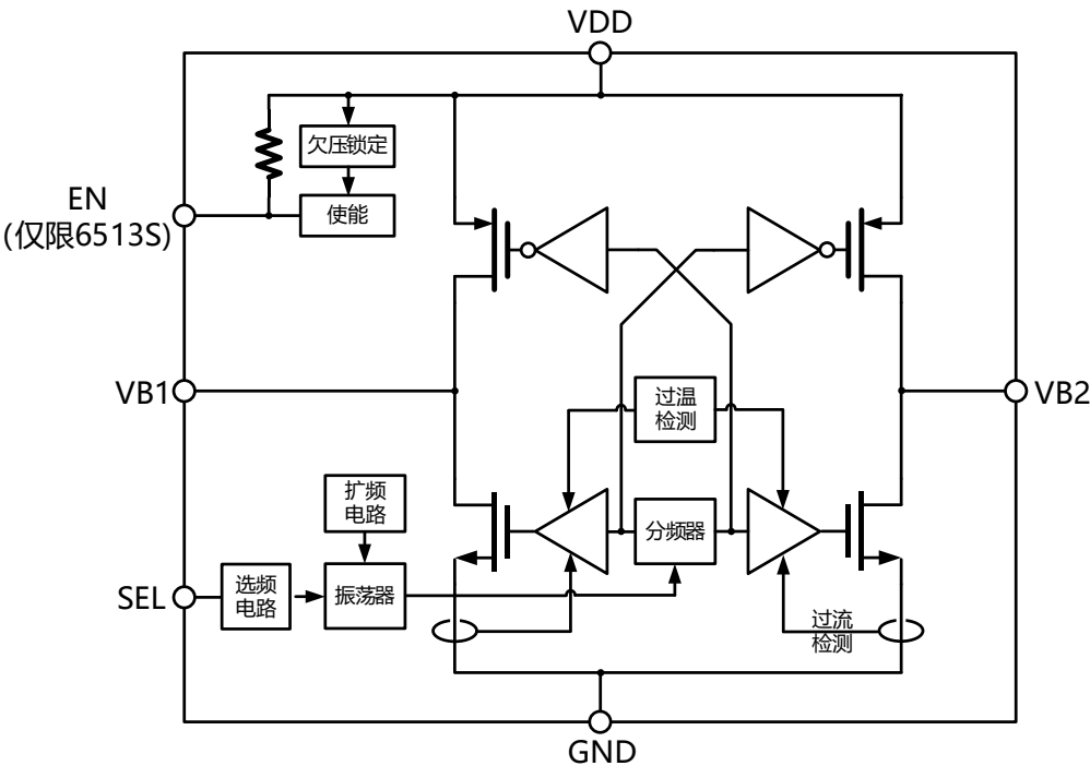
图 7.1 原理示意图
