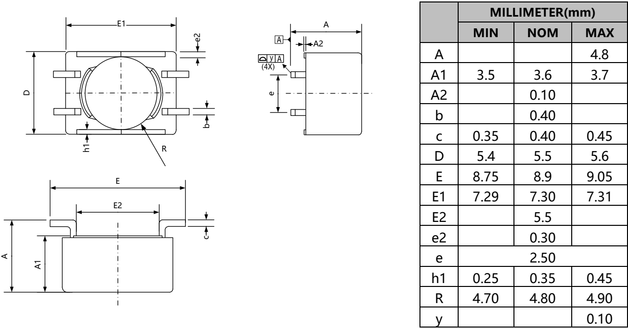
Fig. E.1 SMD-4 器件外形 (所有尺寸单位为 mm)
