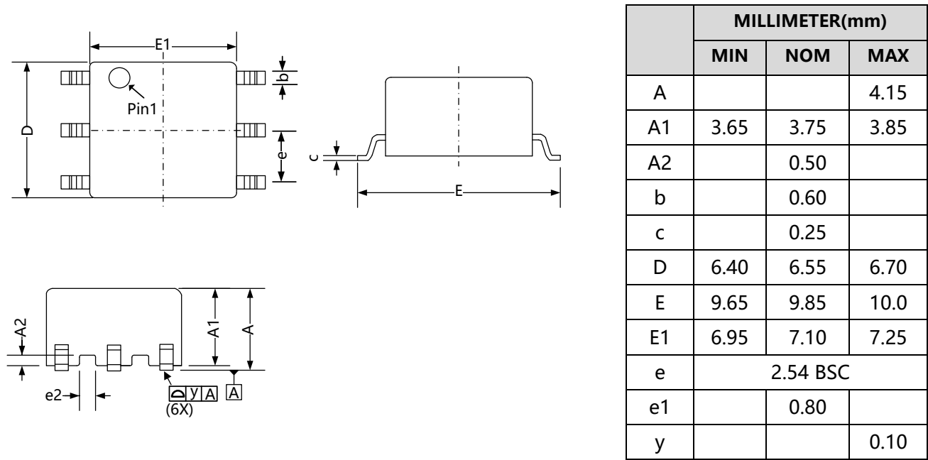
Fig. C.1 SMD-6 器件外形 (所有尺寸单位为 mm)
