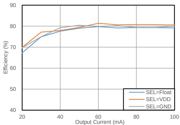
图 8.8 转换效率 vs 输出电流 (CMP6503S+CMT6870N, 3.3V to 3.3V)
