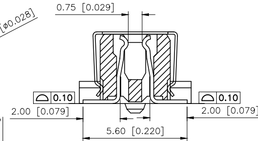
SECTION:A-A SCALE 2:1
