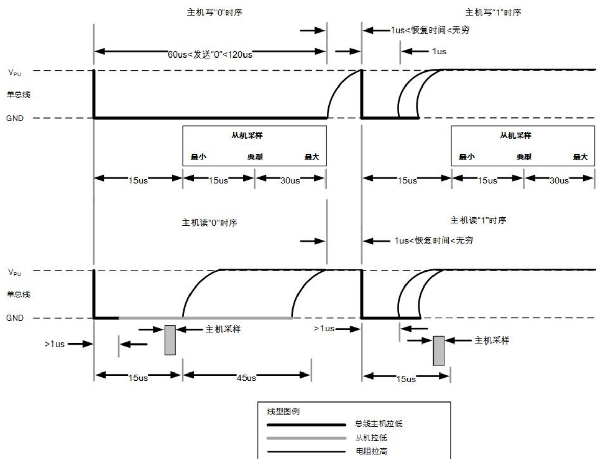
图 11.6-2 读/写时序
