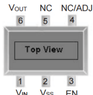
SOT23-6L
