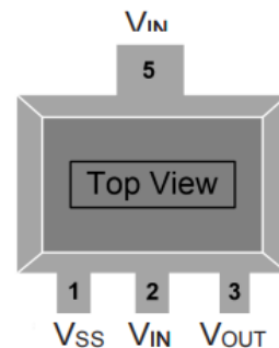
SOT89-3L
