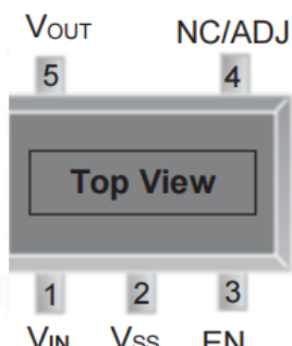
SOT23-5L
