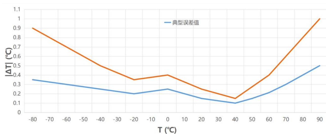
图 7-5 MTS4PF 精度误差曲线
