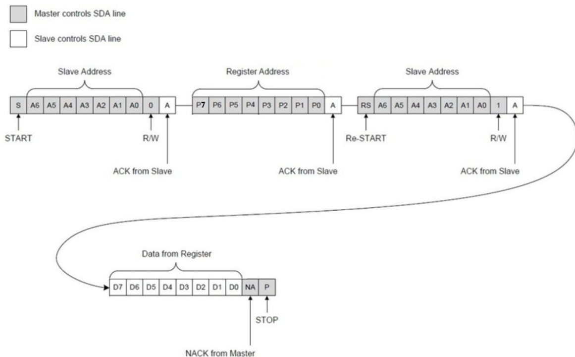
图 11.2-1 I²C 读时序
