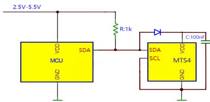
图 9.9-1 寄生模式典型电路图（外接二极管）
