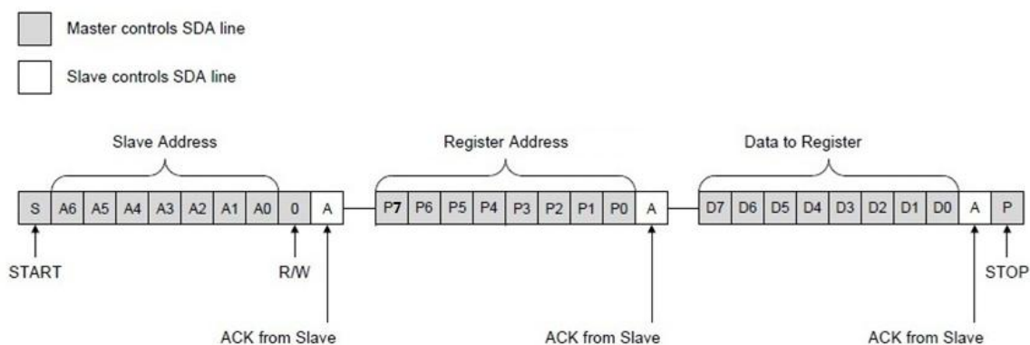
图 11.2-2 I²C 写时序
