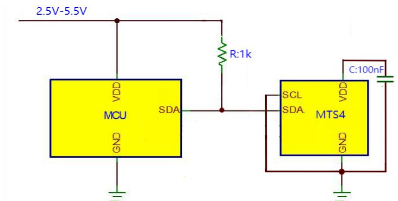
图 9.9-2 寄生模式典型电路图（修改寄存器）
