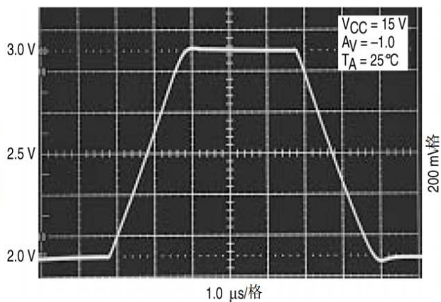
图 4. 误差放大器大信号瞬态响应
