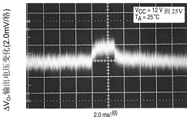
图 10. 参考电源调整率
