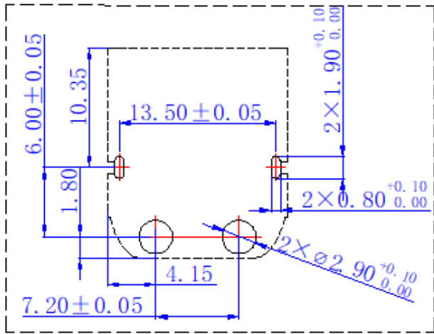
互配尺寸
