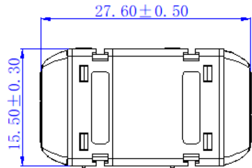
互配尺寸
