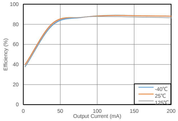
图 7.4 转换效率 vs 输出电流
