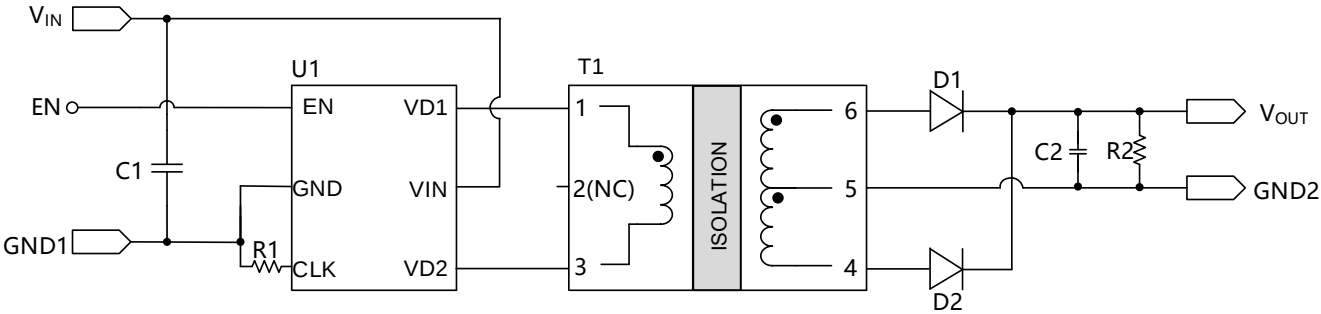
图 9.1 设计原理图
