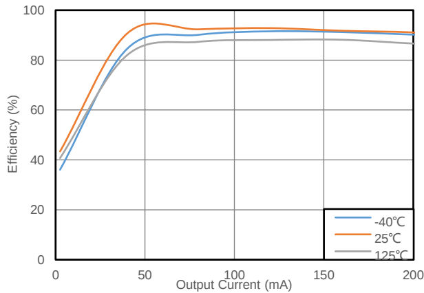
图 7.3 输出电压 vs 输出电流
