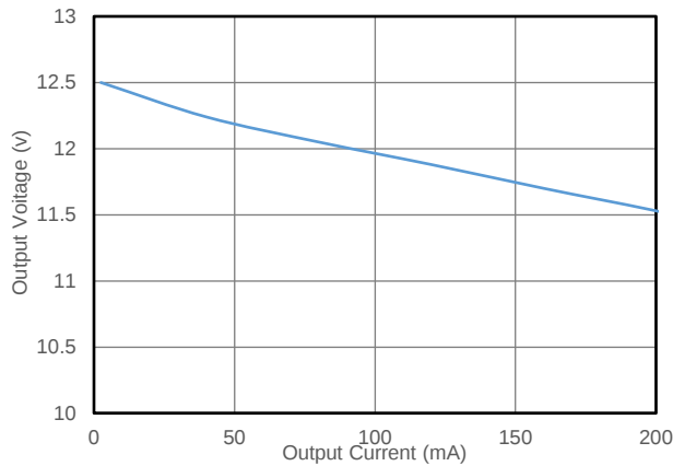
图 7.1 输出电压 vs 输出电流
