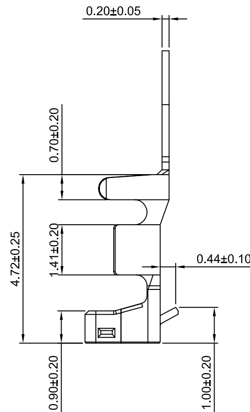
SEC:B-B
