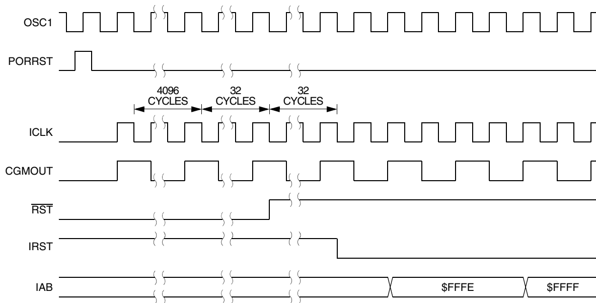
Figure 9-7. POR Recovery
