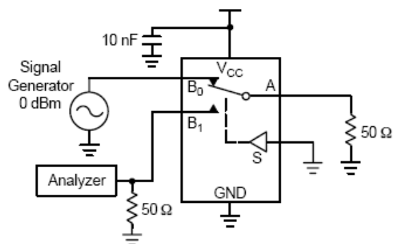
图 5 串扰
