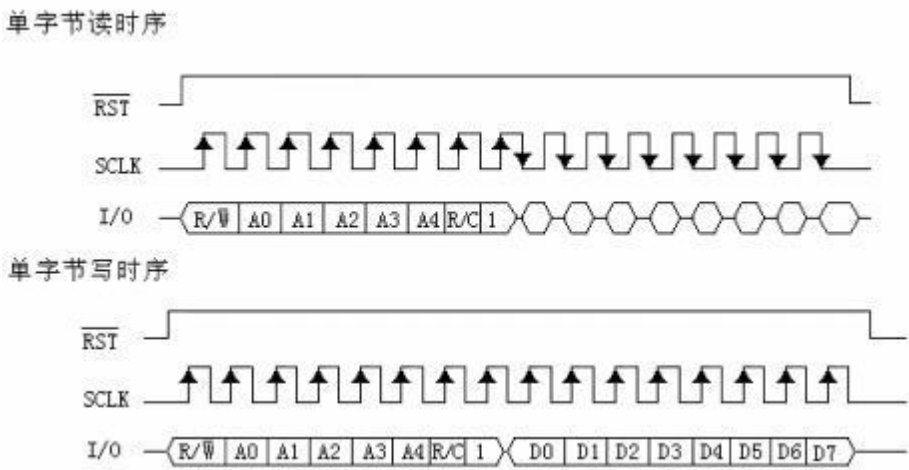
图 3 DS1302ZN数据传送图示
