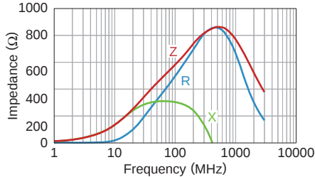
MMZ1005A601ET000
