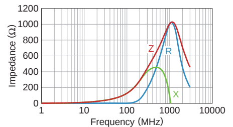
MMZ1005F750ET000
