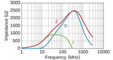
MMZ1005A152ET000
