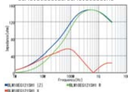
BLM18EG121SZ1/BLM18EG121SH1
