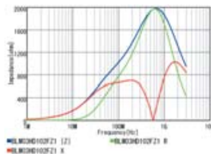
BLM03HD102FZ1
