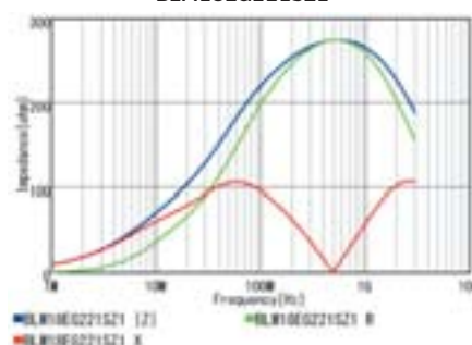
BLM18EG221SZ1
