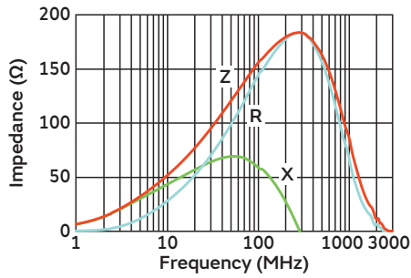
BLL18AG151A2E1H01/BLL18AG151DBE1H01
