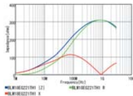
BLM18EG221TZ1/BLM18EG221TH1
