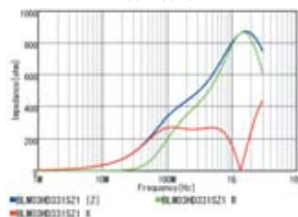
BLM03HD331SZ1
