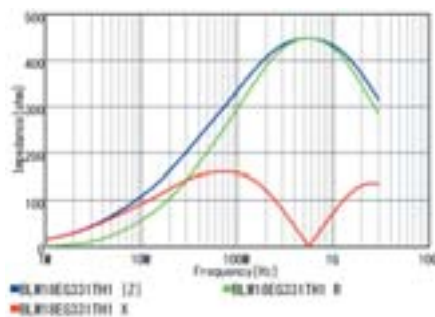
BLM18EG331TZ1/BLM18EG331TH1
