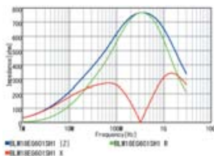
BLM18EG601SZ1/BLM18EG601SH1
