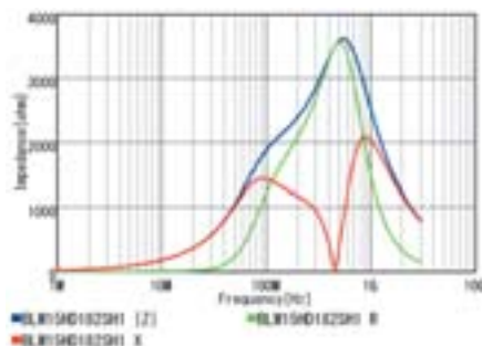
BLM15HD182SZ1/BLM15HD182SH1
