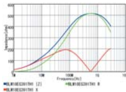
BLM18EG391TZ1/BLM18EG391TH1
