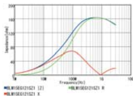
BLM15EG121SZ1/BLM15EG121SH1
