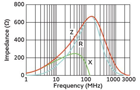
BLL18AG601A2E1H01/BLL18AG601DBE1H01
