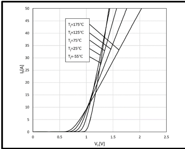
图 1 典型正向特性曲线
