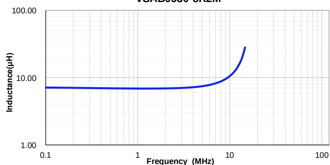
VSAB0630-8R2M
