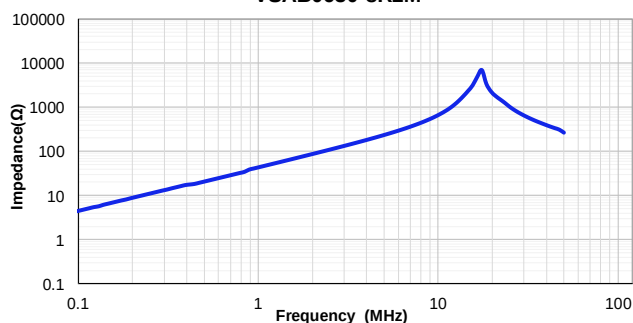
VSAB0630-8R2M
