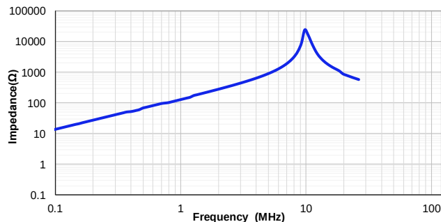
VSAB0630-220M
