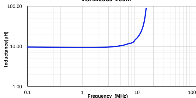
VSAB0630-100M
