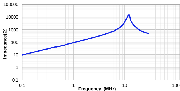
VSAB0630-150M
