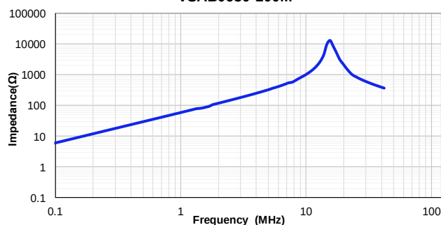
VSAB0630-100M
