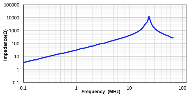
VSAB0630-5R6M
