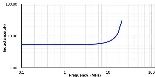
VSAB0630-5R6M
