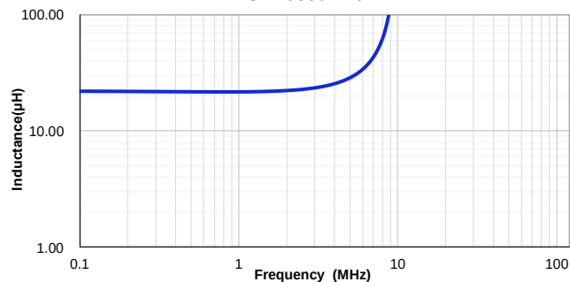
VSAB0630-220M
