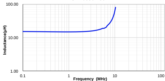
VSAB0630-150M
