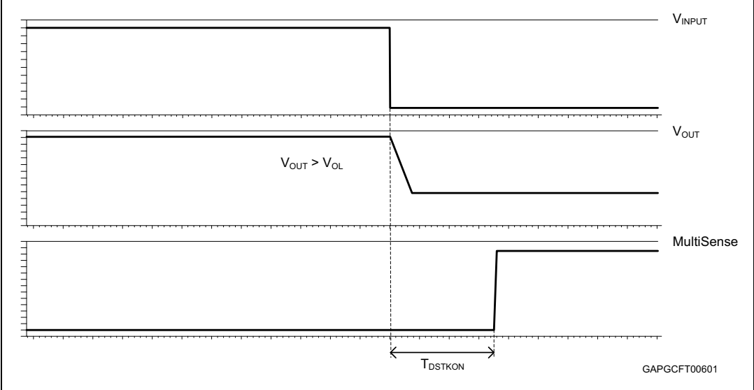
Figure 9. T_{DSTKON}
