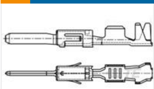
TE Part #963904-3 TAB A 1.6x0.6 CONTACT CS SWS Au
