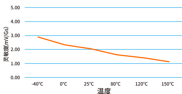
1.8V下灵敏度温度特性曲线
