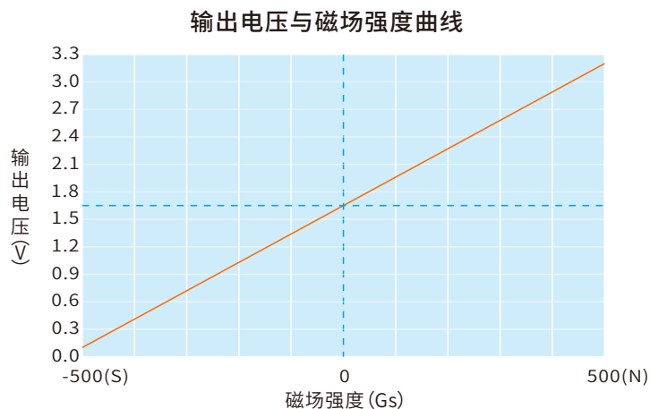
HAL403 SOT-23示例图
