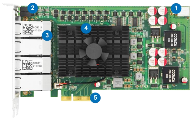
产品布局图
