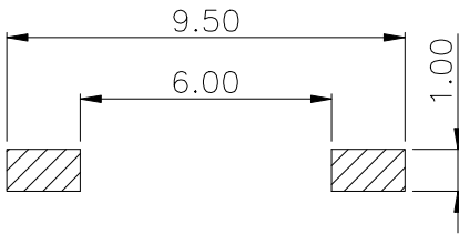
PCB.焊接图
