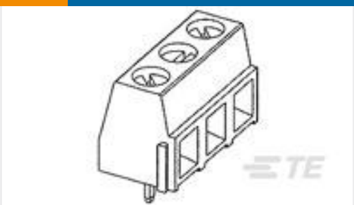
TE Part #NB15964001 RT-375-1/4-X-SP
