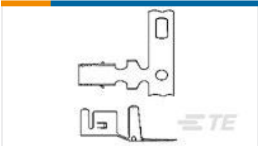
TE Part #3-770060-1 MINI AMP-IN PTL/PHBZ
