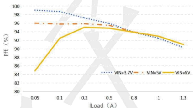
Eff.—3.3V Output
