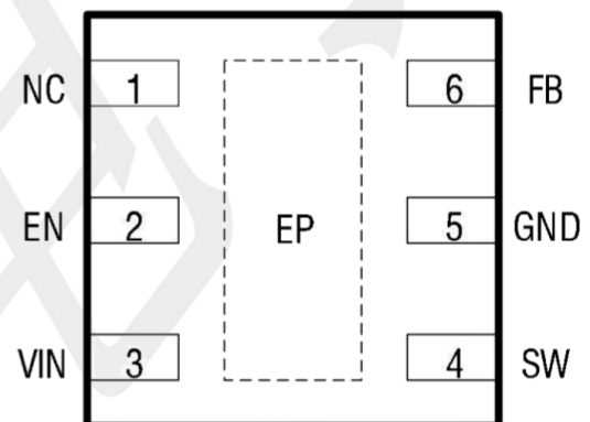
DFN-6(2X2)
