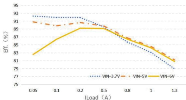
Eff.—1.2V Output
