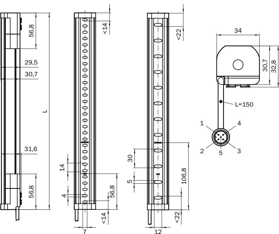
尺寸图 (尺寸单位: mm)
