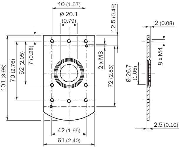
尺寸图 (尺寸单位: mm)
