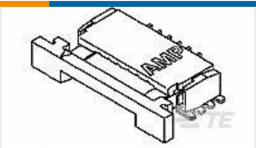
TE Part # 1-487952-1 011 1MM FPC BTM HORZ
