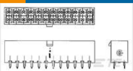
TE Part #1-1586038-0 10P VRT HDR VAL-U-LOK V0
